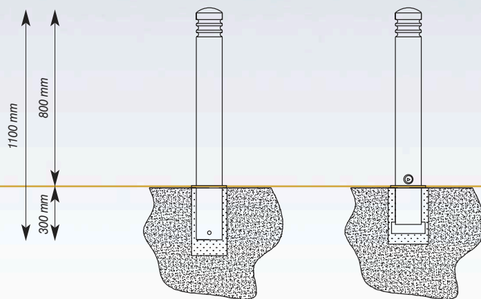
Montaż do podłoża przez zabetonowanie rury kotwiącej
